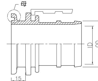
插管(20kg/cm 2 )
