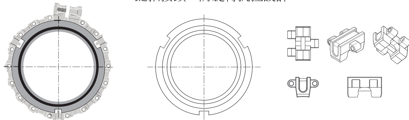
鏈扣接頭—防旋轉抗拉設計
