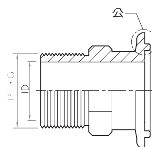
轉接頭
